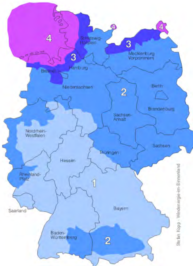
Abbildung 50: Windzonen in Deutschland nach DIN 1055-4:2005-03 (Windenergie 2019)
